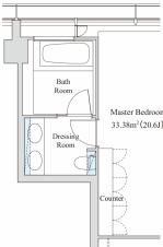
■33F部分図
